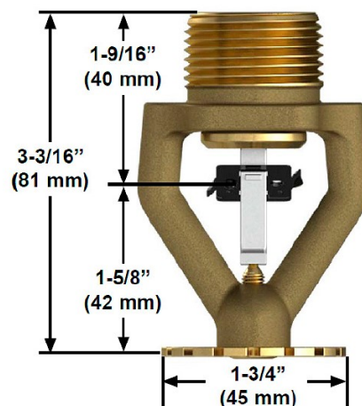
Рис 2 Размеры спринклера ESFR VK510
